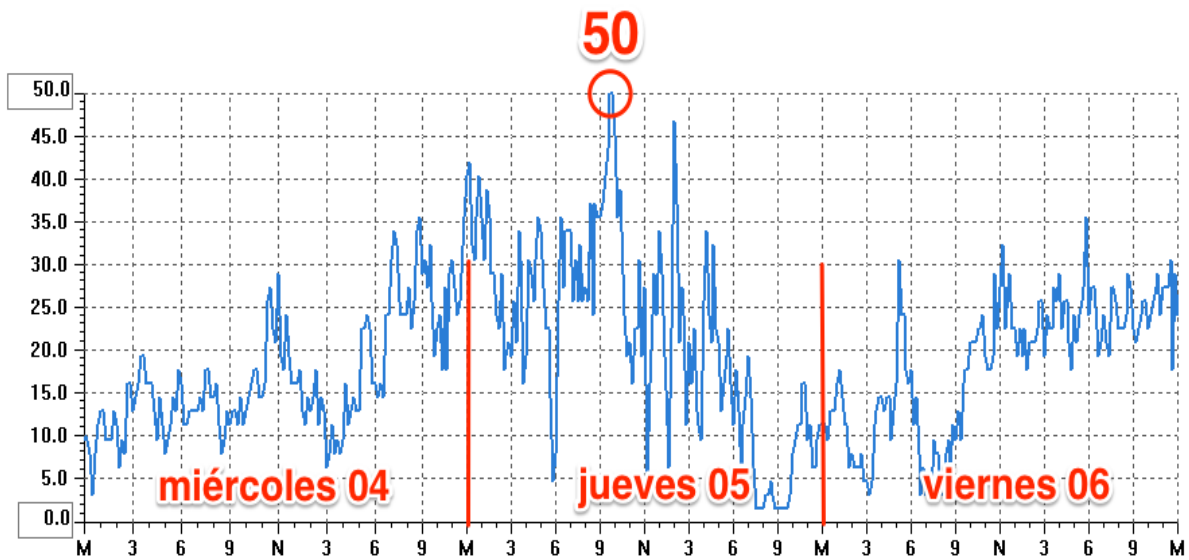
Ráfagas de viento registradas en ALZIRA (estación "Est-Alquenència") entre el 04 y el 06/11/20 (en km/h)
