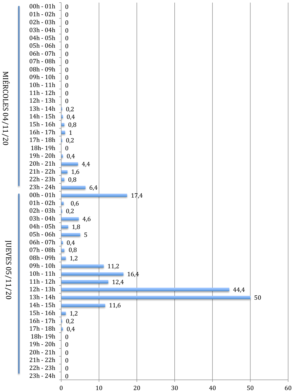
Cantidades de lluvia registradas por horas en ALZIRA (estac. "Ajuntament") los días 04 y 05/11/20 (en l/m²)
