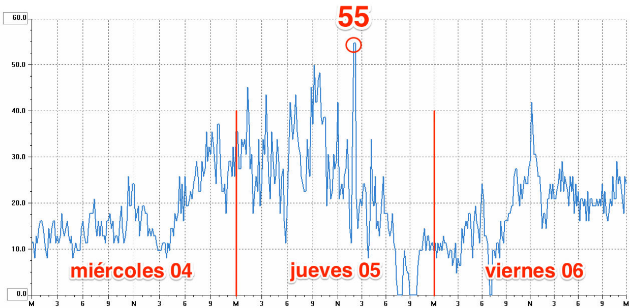
Ráfagas de viento registradas en ALZIRA (estación "Ajuntament") entre el 04 y el 06/11/20 (en km/h)
