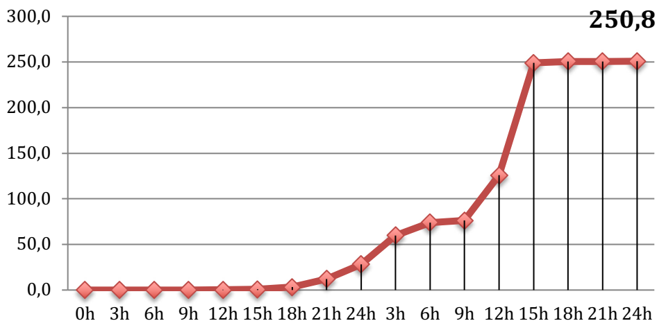
Evolución lluvia acumulada en ALZIRA (Est-Alquenencia) los días 04 y 05/11/20 en períodos de 3 horas (en l/m 2 )
